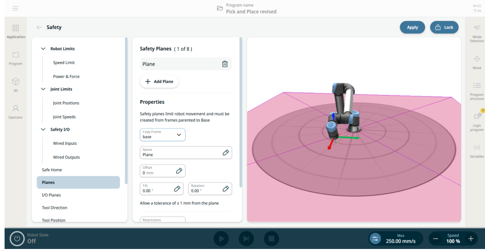
Çizim 1.5: Güvenlik düzlemlerini gösteren PolyScope X ekranı.
