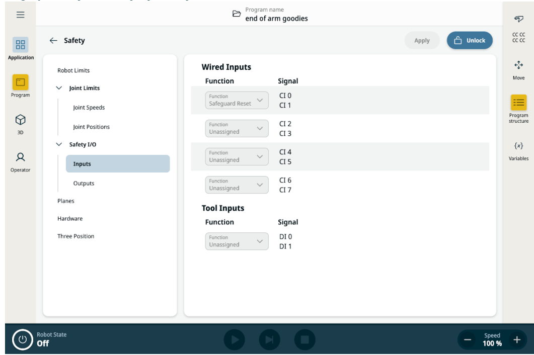
Çizim 1.4: PolyScope X ekranında Giriş sinyalleri gösterilir.
