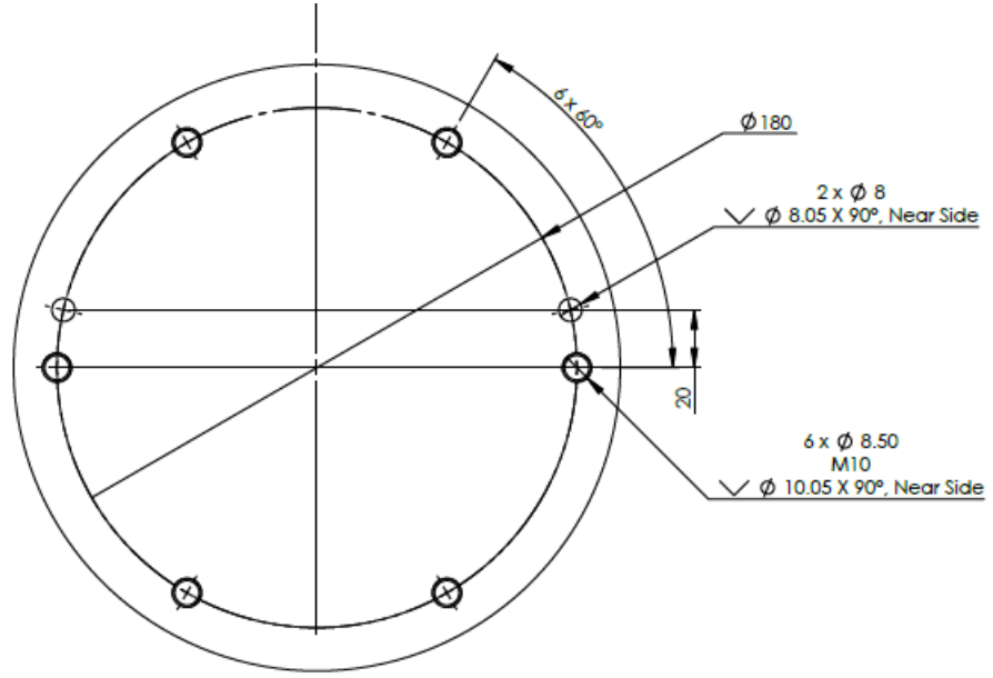
1.1: Robot tabanının alttan görünümü
