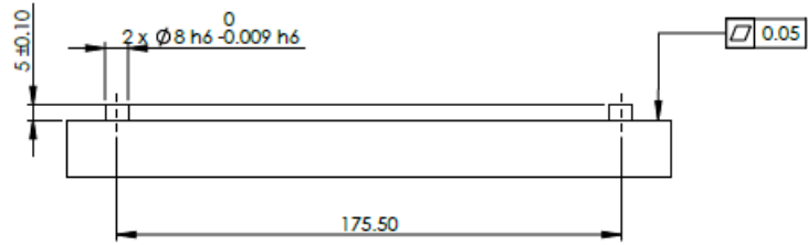
1.2: Robot tabanı için montaj plakası
